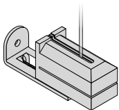
Klemmträger für Seilführung Klemmbereich 5–25 mm
